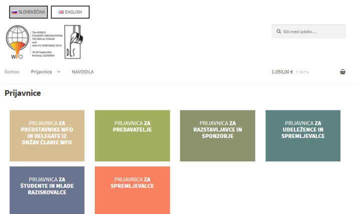
Slika 1: Vrste prijavnic
