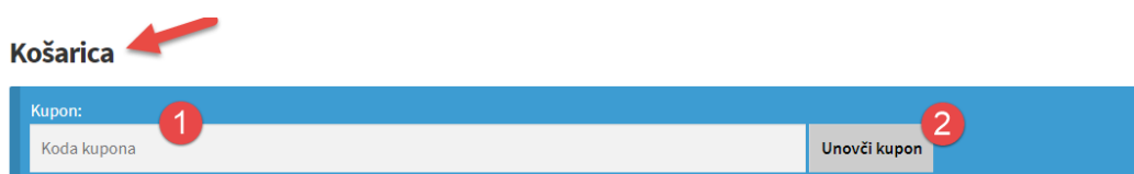
Slika 8: Koda kupona
